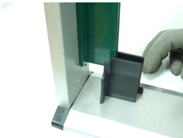
7 Inserimento piedino con unico foro
